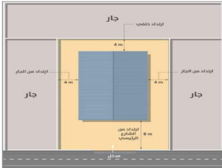
مثال (أ) يوضح الارتدادات لموقع مستقل ومناطق الخدمات المساندة
