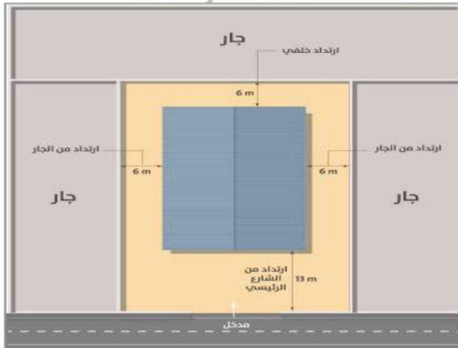
مثال (ب) يوضح الارتدادات في المواقع المعتمدة كمخططات للمصانع
